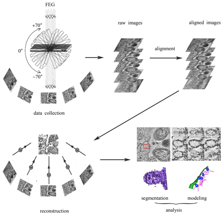
图 3 电子断层三维重构技术原理和流程示意图 以猪动脉内皮细胞胞膜容电子断层三维重构 [39] 为例，其技术路线主要包括：从各个投影角度收集原始图像，图像的匹配和归一化，空间几何参数的确定，三维重构，数据后处理，数据分析（密度分割和建模等）
