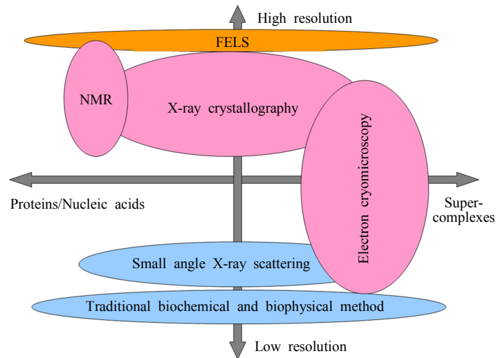
图 1 结构生物学各种研究手段的比较 纵轴表示分辨率（从下向上，分辨率逐渐升高），横轴表示研究尺度（从左至右，尺度逐渐增大）。小角散射（small angle X-ray scattering）和众多传统生物物理生物化学技术（traditional biochemical and biophysical method）能够适于研究各种尺度的生物分子，但分辨率信息较低；核磁共振技术（NMR）的解析分辨率较高，但是研究尺度较小；X 射线晶体学（X-ray Crystallography）的研究尺度范围较宽，并能得到较高分辨率的结构（多数情况下可以得到原子分辨率），然而其瓶颈是需要结晶；冷冻电镜技术（cryo-electron microscopy）可以获得超大分子复合物的三维结构，并一般能达到中等分辨率（纳米级）；自由电子激光散射技术（free electron laser scattering, FELs）是目前正在发展的技术，有望能够在多种尺度上获得生物大分子的接近原子分辨率的三维结构
